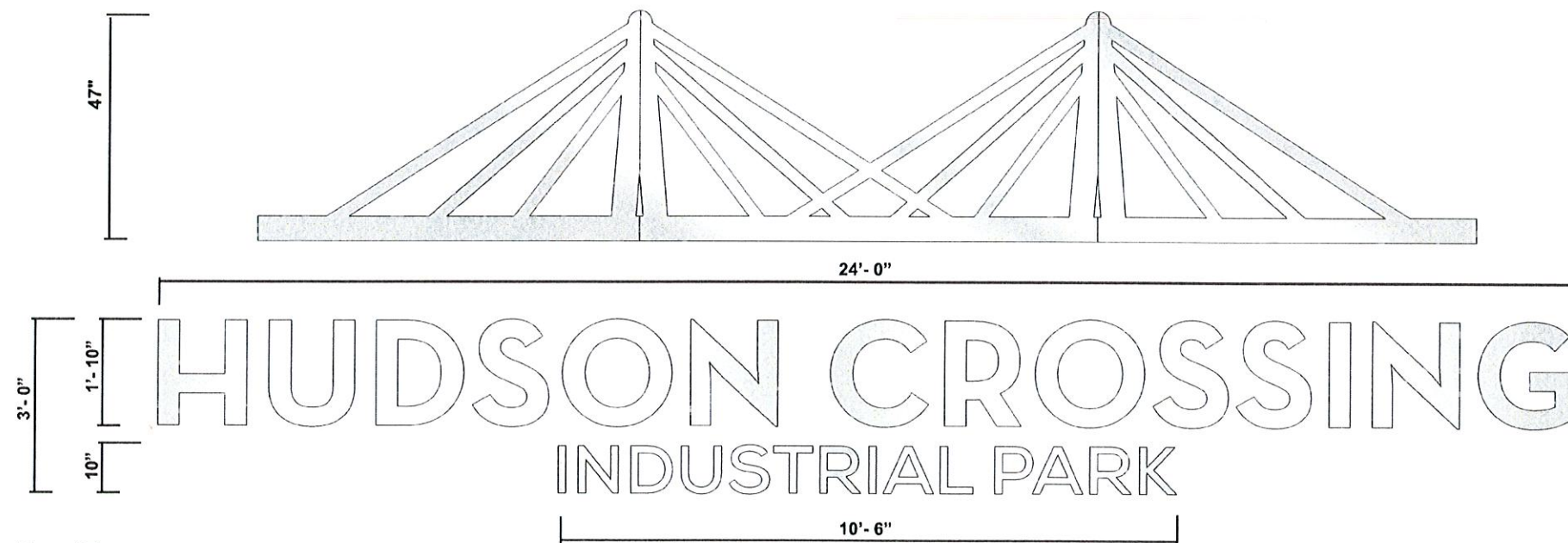
Face View Scale: 3/8" = 1' - 0"
